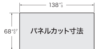
AD-8923-CC/BCD共通寸法
