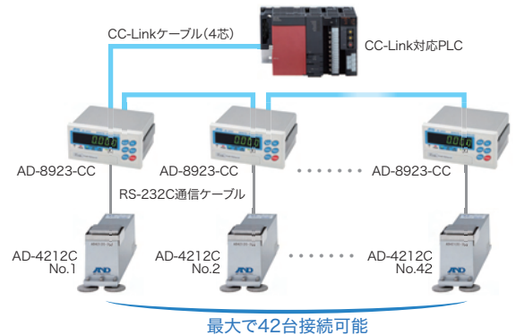
AD-8923 (CC-Link接続) を利用した計量ライン用システム
