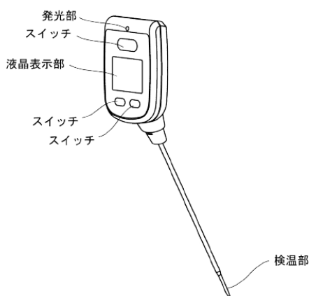
【各部の名称を示す参考正面斜視図】
