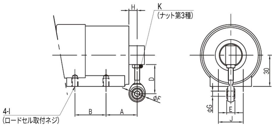
U2Z1シリーズ着図イメージ
