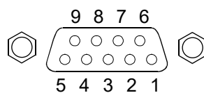
拡張端子 1
