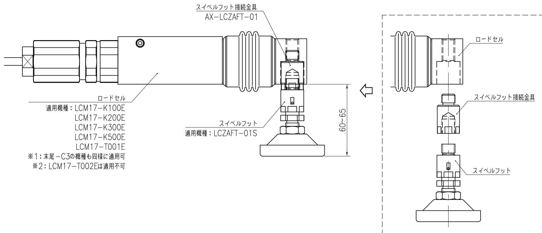
装着図
