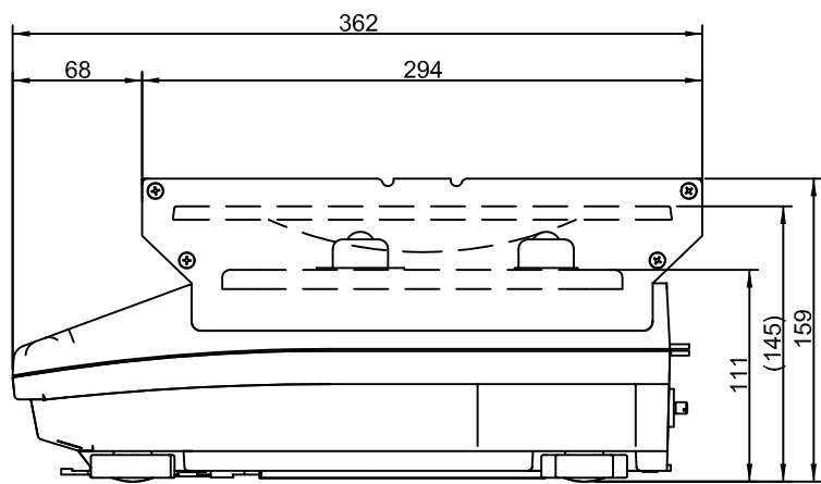
MC10K/30K 重心調整皿外観図
