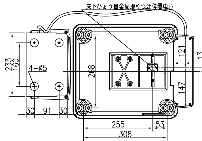
裏面寸法
