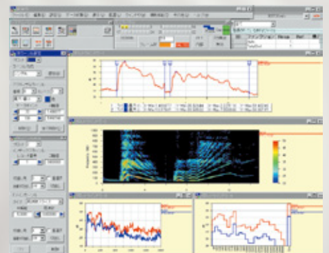
過渡騒音計測
