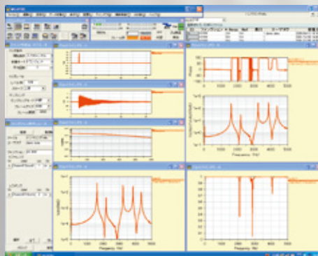
伝達関数測定
