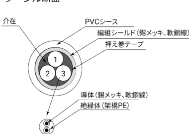
ケーブル断面
