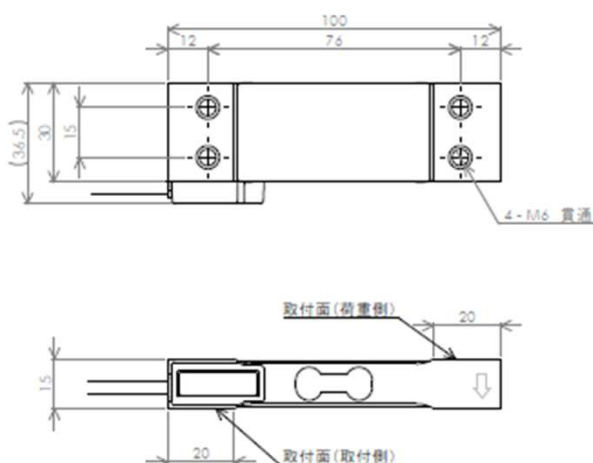
外形寸法図
