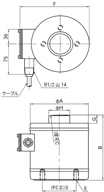
外形寸法図
