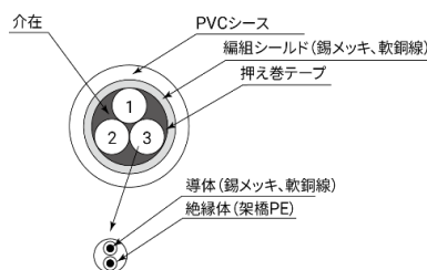
ケーブル断面
