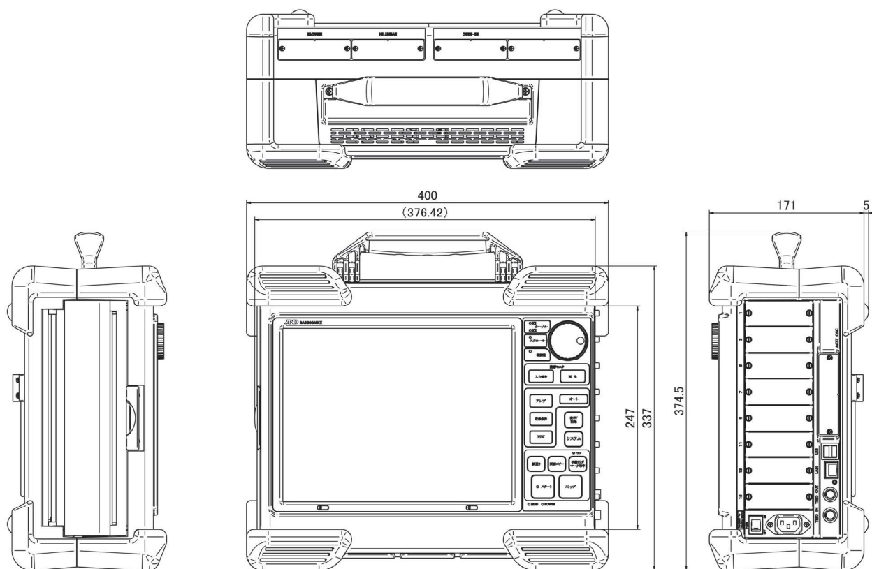
■ RA2300MKII(-S)外形図
