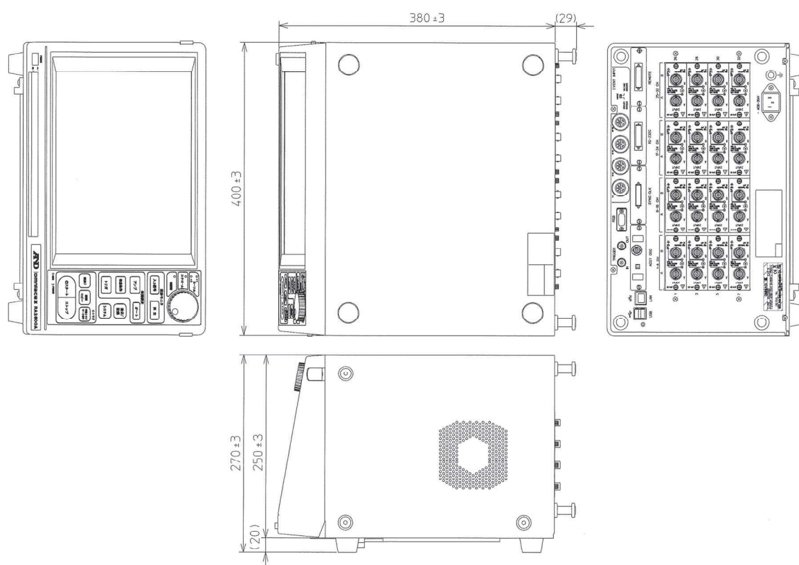
■ RA2800A外形図
