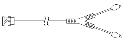
信号ケーブル AS30-503 (金属 BNC ⇄ ミノ虫 (十…赤、一…黒)、長さ 2m)
