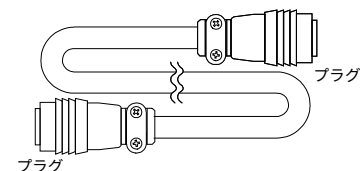
中継ケーブル AS30-501-xxx (φ9.6mm、4芯シールド、長さ xxx=1、2、5、10、15、20、25mあり)
