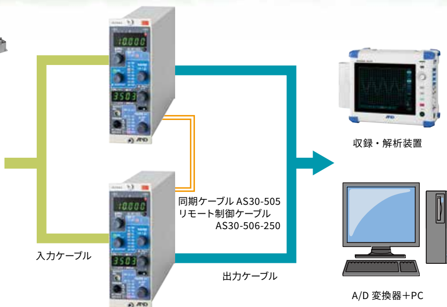
ひずみゲージ + ブリッジボックス
