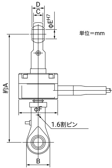
■装着図 UM
