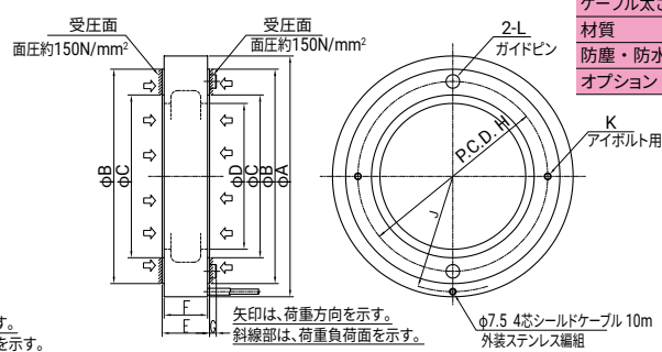
RWL-100~500
