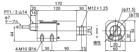
U2Z1-200L-A, 500L-A
