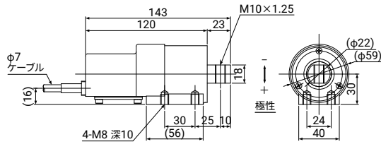
U2Z1-200L-A, 500L-A
