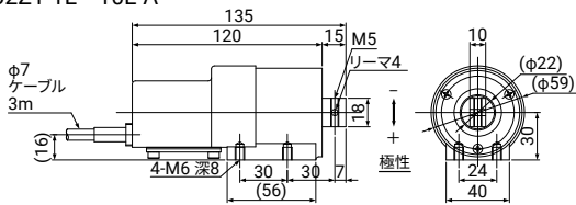
U2Z1-20L~100L-A
