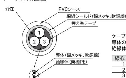
ケーブル断面図
