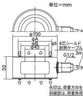
RWL-10~50
