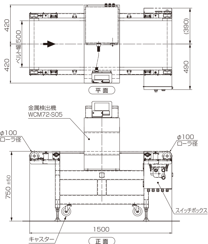
WCM72-S05 外観図
