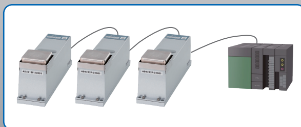
自由自在なレイアウト (RS-485 デイジーチェーン接続例)
