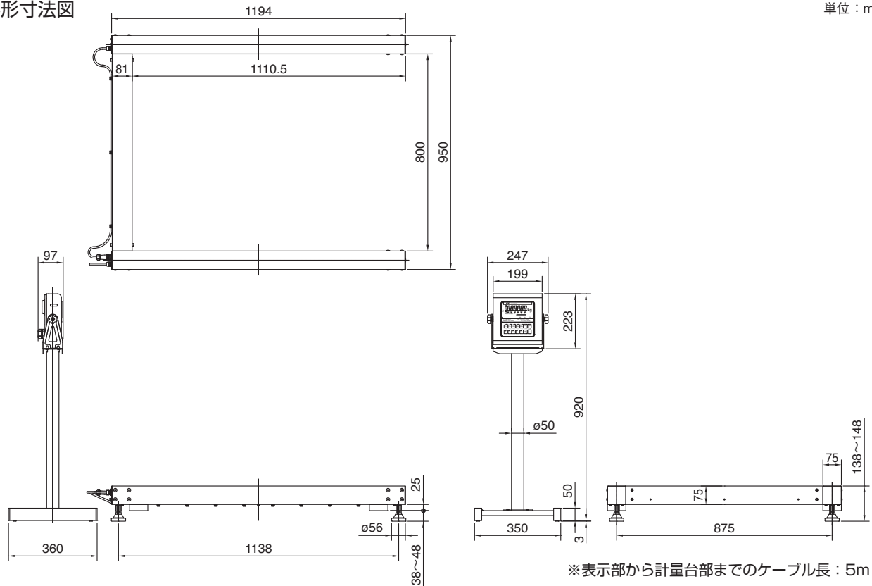
外形寸法図
