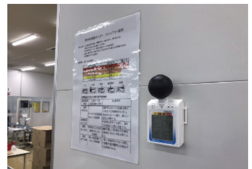
工場内の随所に説明書きと合わせて設置されている、 A&D製熱中症指数計 みはりん坊プロAD-5698
