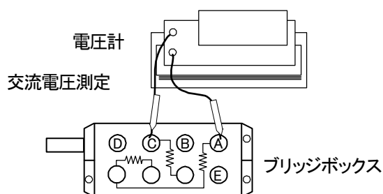
図4-11 1ブリッジ部の電圧測定
