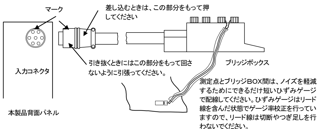
図3-1 ブリッジボックスとの接続
