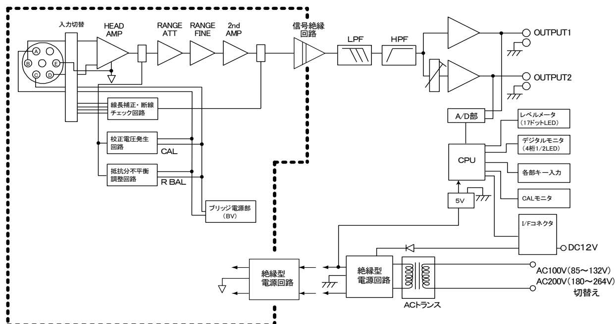
図5-1 AS2503 ブロック図
