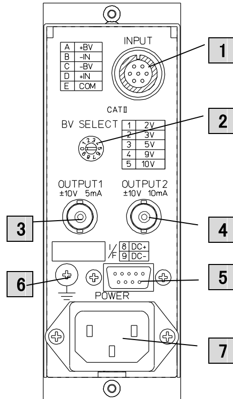
図2-2 : AS本体背面
