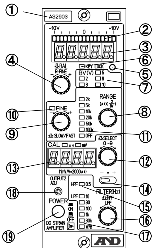
図 2-1 : AS 本体正面 (図は AS 2603)
