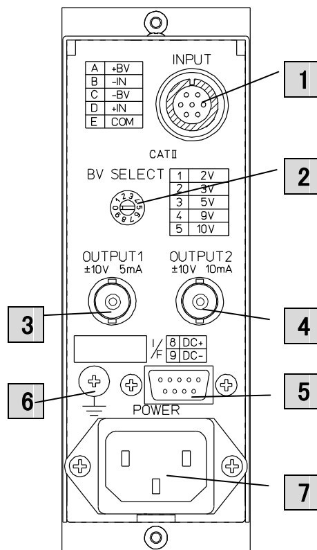
図 2-2 : AS 本体背面
