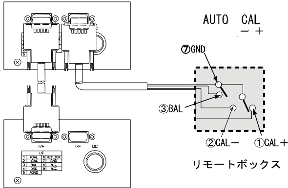
図3-10 リモートボックスの概略図
