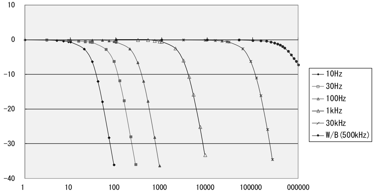
AS2503 周波数特
