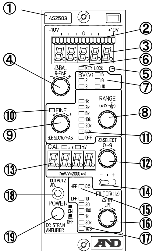
図2-1 : AS本体前面 (図はAS2503)
