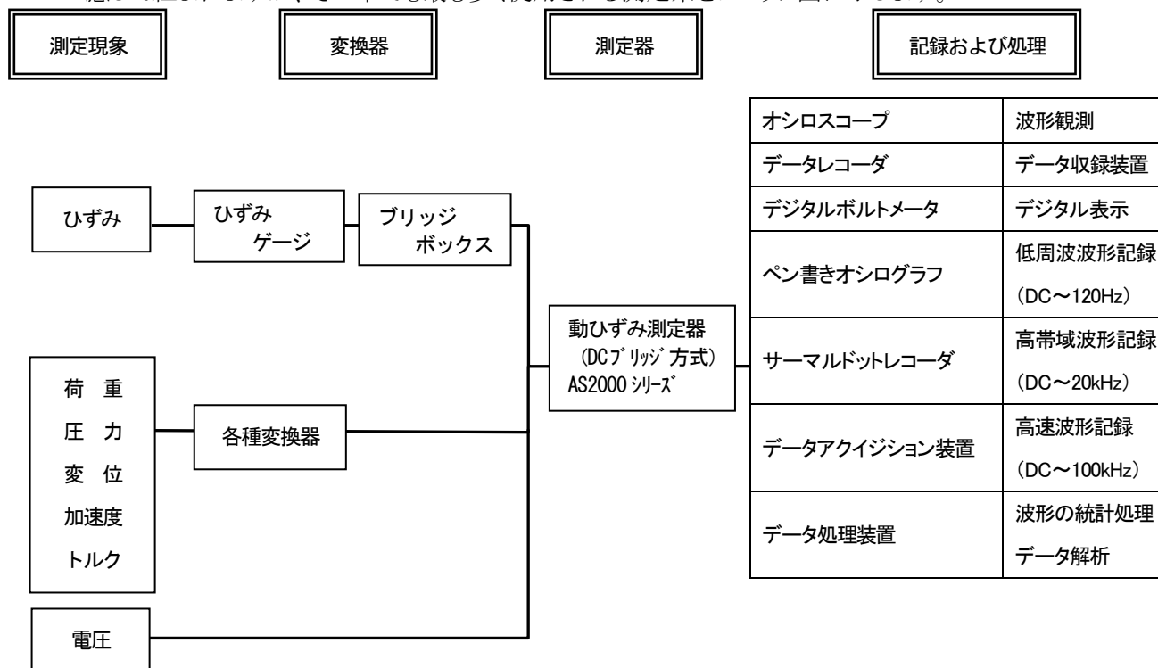
図 1-1 計測ブロック図 1-2
