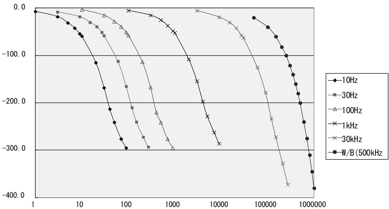
AS2503 位相特性
