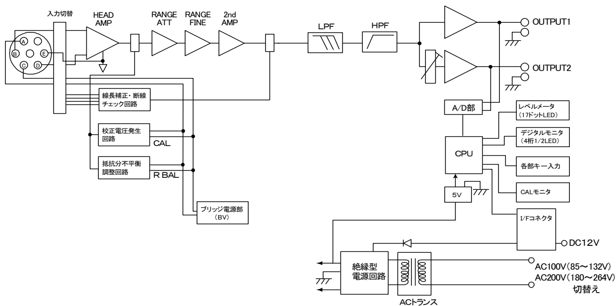
図5-1 AS2503 ブロック図
