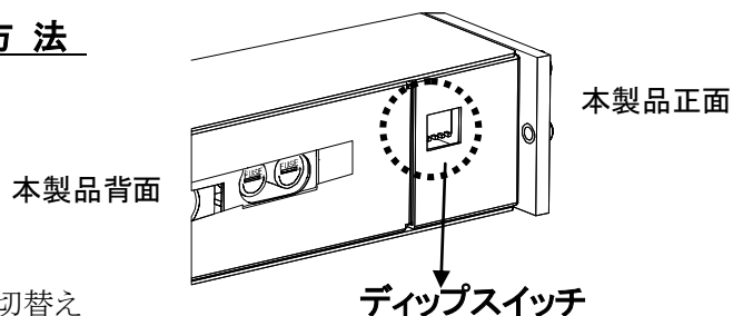
図3-6 ディップスイッチの位置
