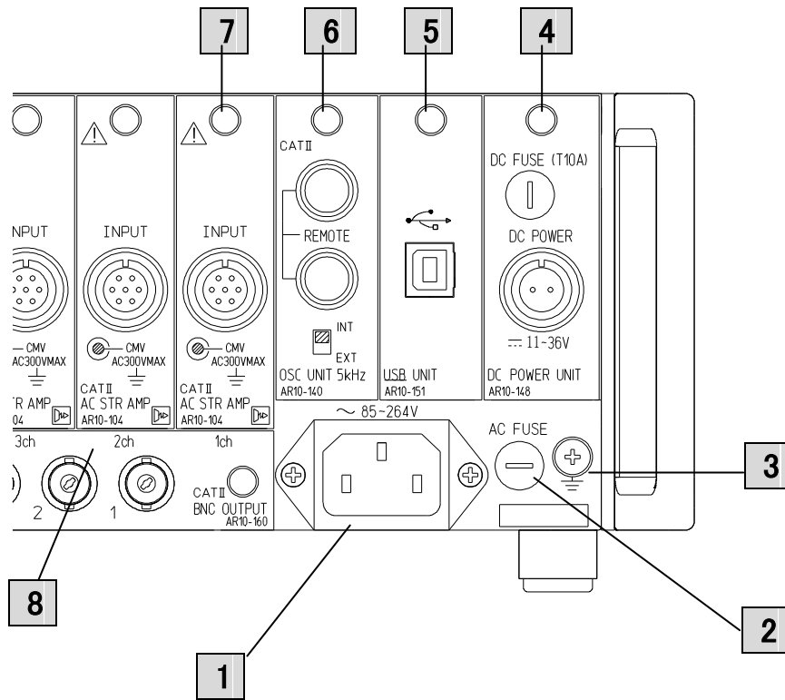
図2-6: 本体背面
