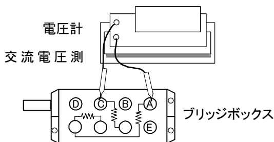
図4-7 ブリッジ部の電圧測定
