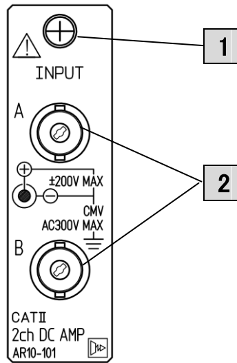
図2-5:2ch DCアンプ入力コネクタパネル
