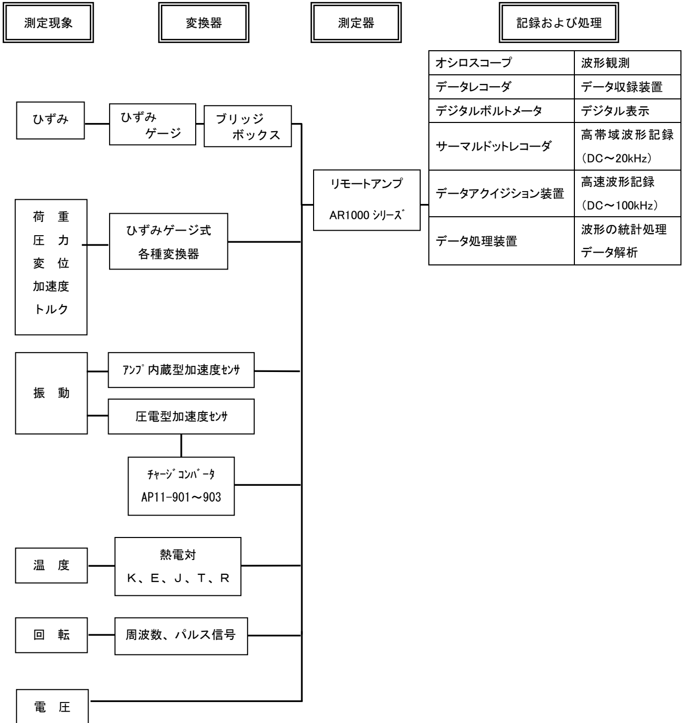
図1-2 計測ブロック図
