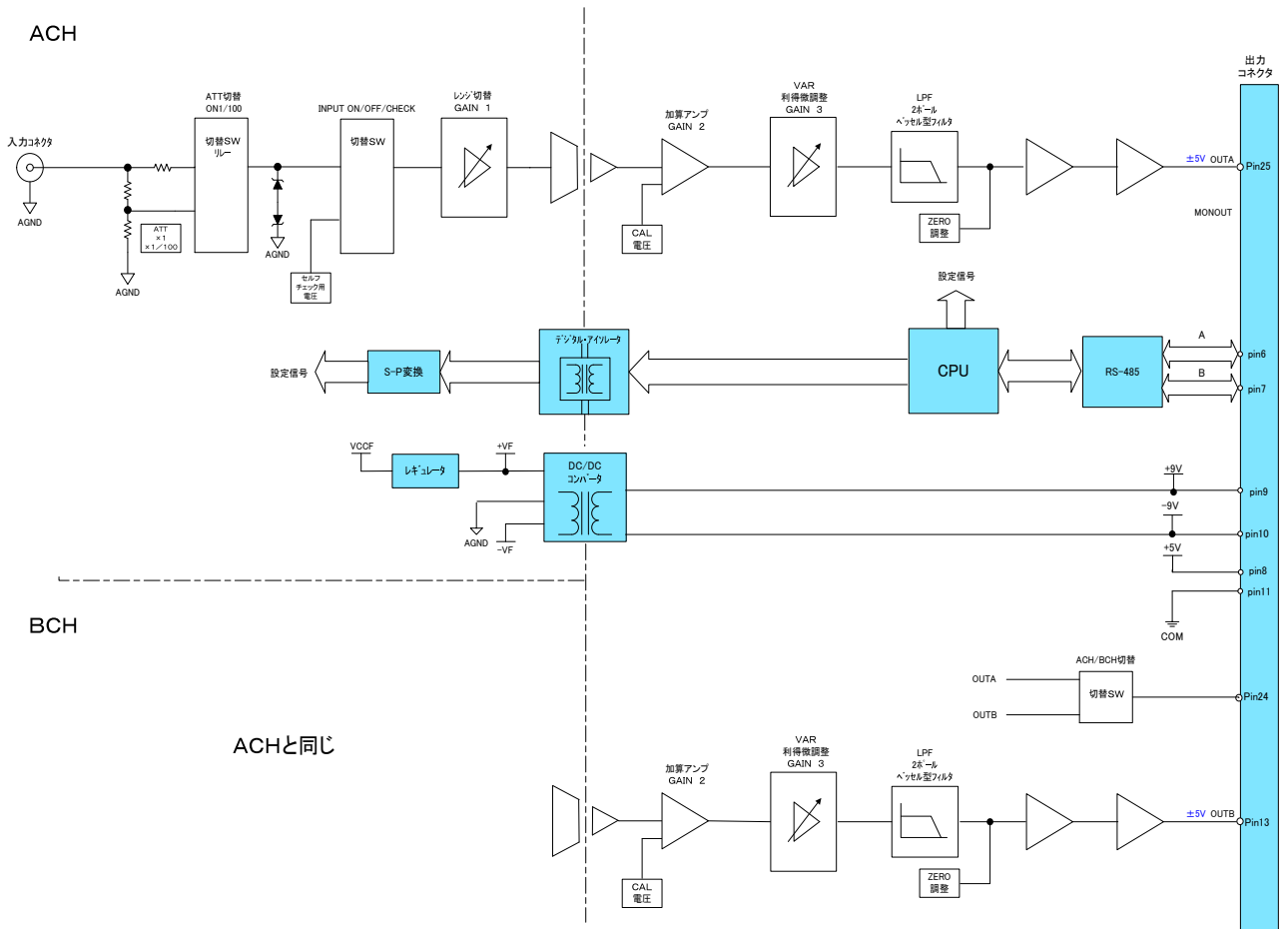
図5-1 ブロック図
