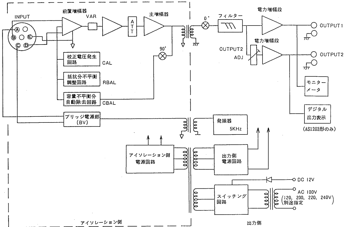
図 23 ブロック図
