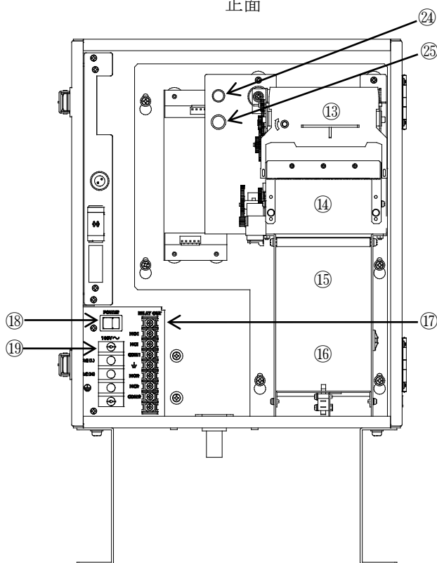
筐体内部
